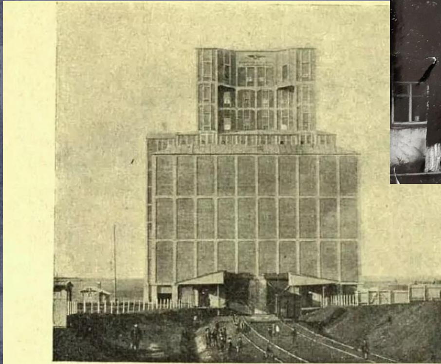
Железобетонный элеватор на ст. Миллерово, Юго-Востоци. н. д., построенный в 1913—1914 г. г.
